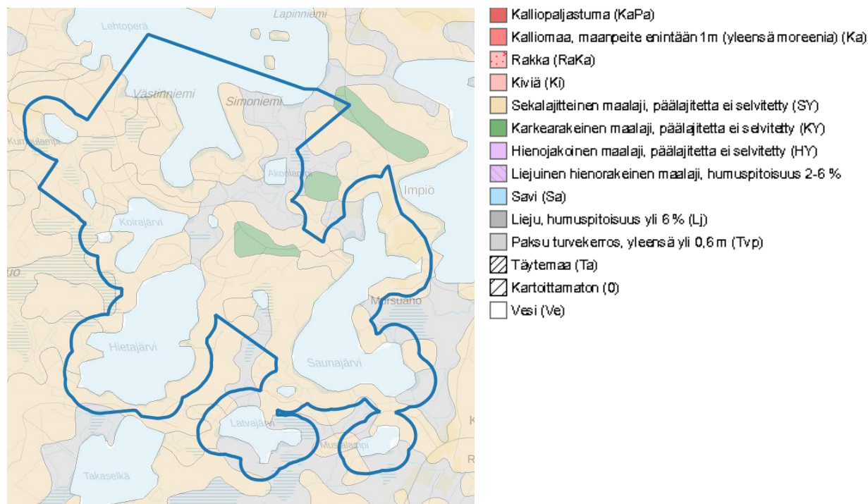
Kuva 11. Maaperä suunnittelualueella.
